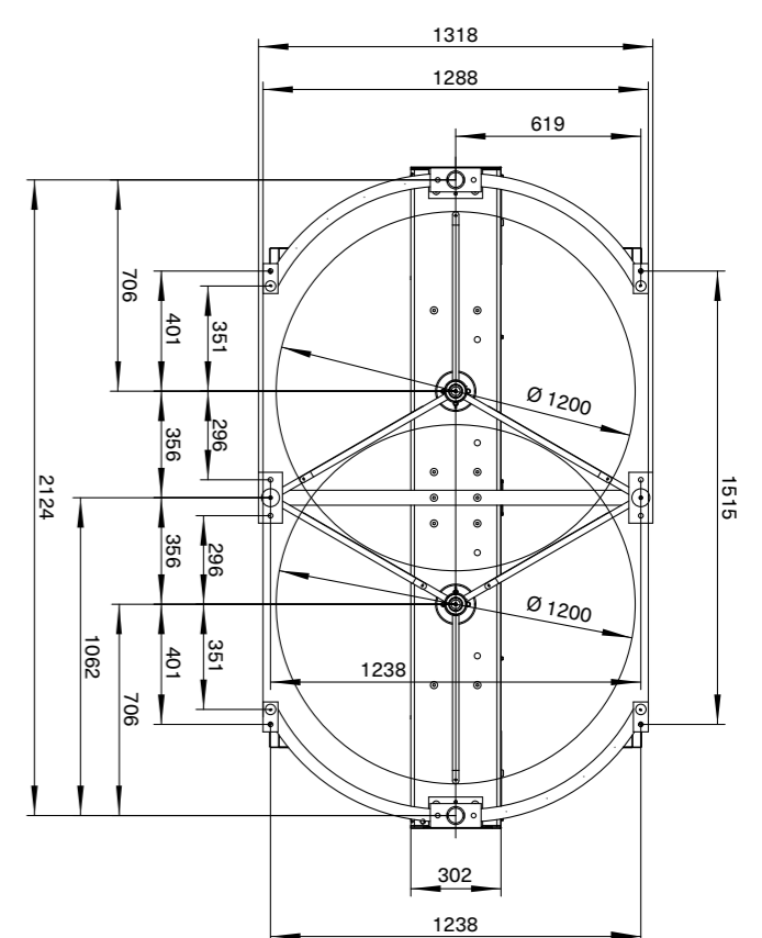
MPT 152/53/50 – 3-flügelige Variante Ansicht von unten
