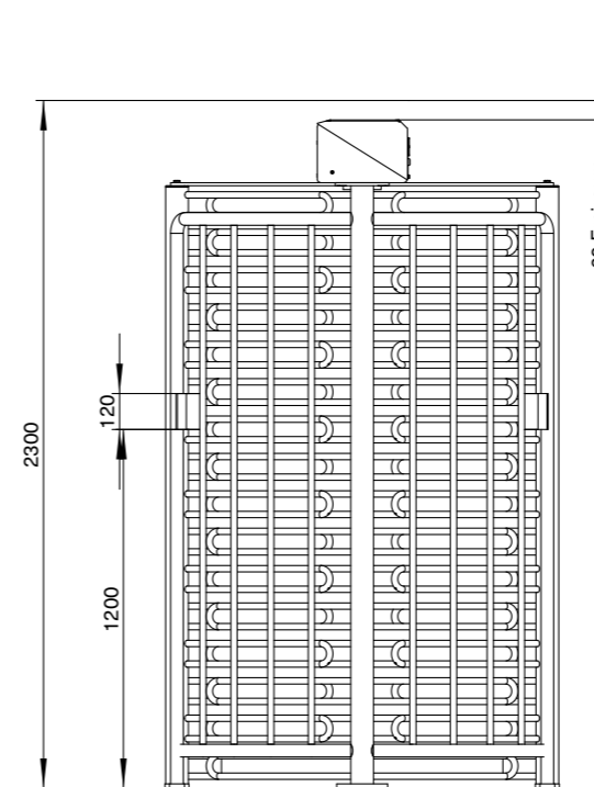
MPT 152/53/50 – 3-flügelige Variante Ansicht von der Seite
